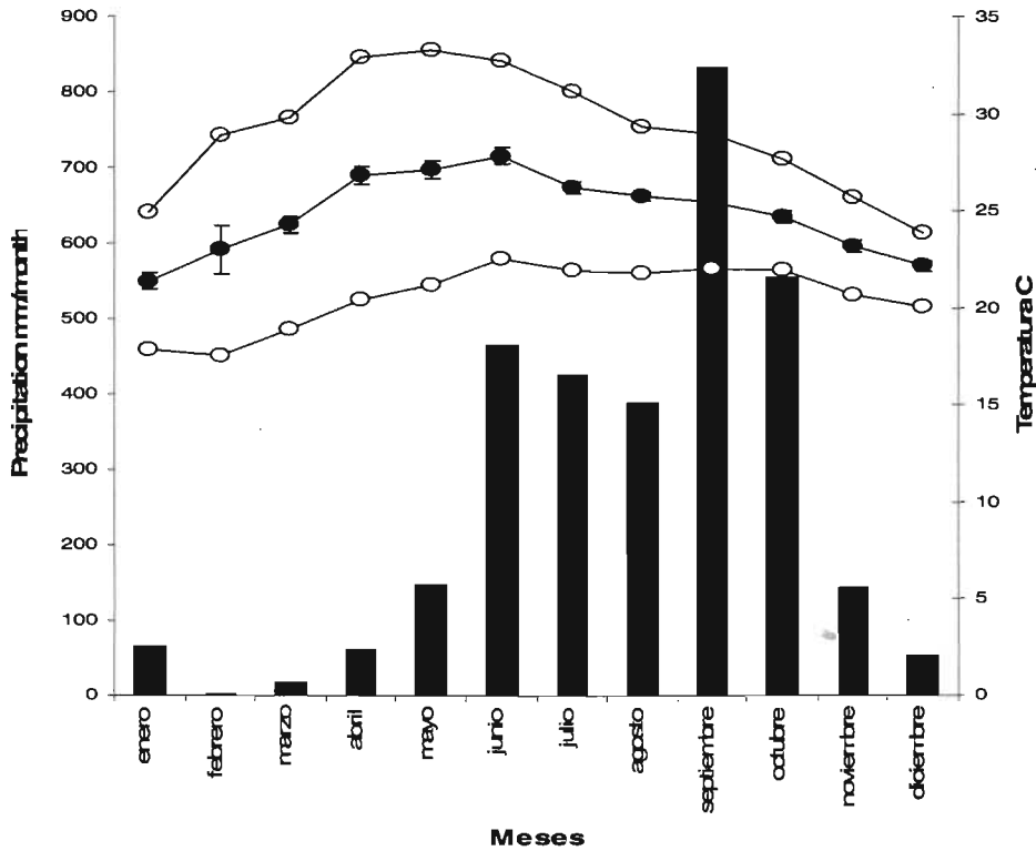
Figura 2. Variación de la precipitación y temperatura promedio mensual de la región de estudio, para el periodo de marzo de 1999 a marzo de 2000 (datos de la Comisión Federal de Electricidad situada en el ejido de Playón de la Gloria).
